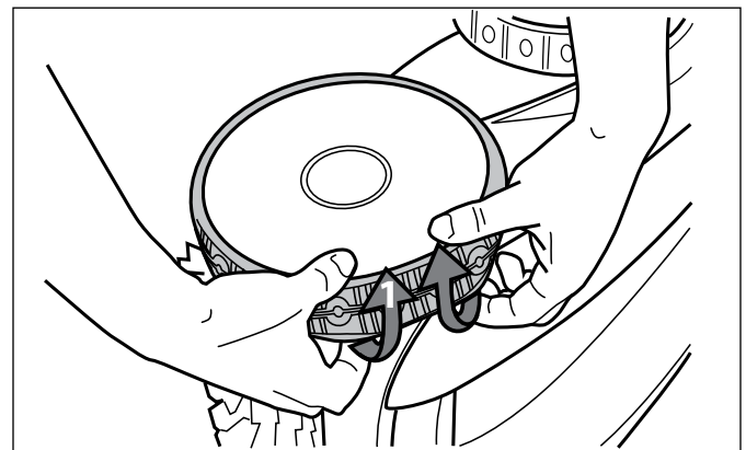
Figure 35. Démontier le pneu utilisé de la roue
