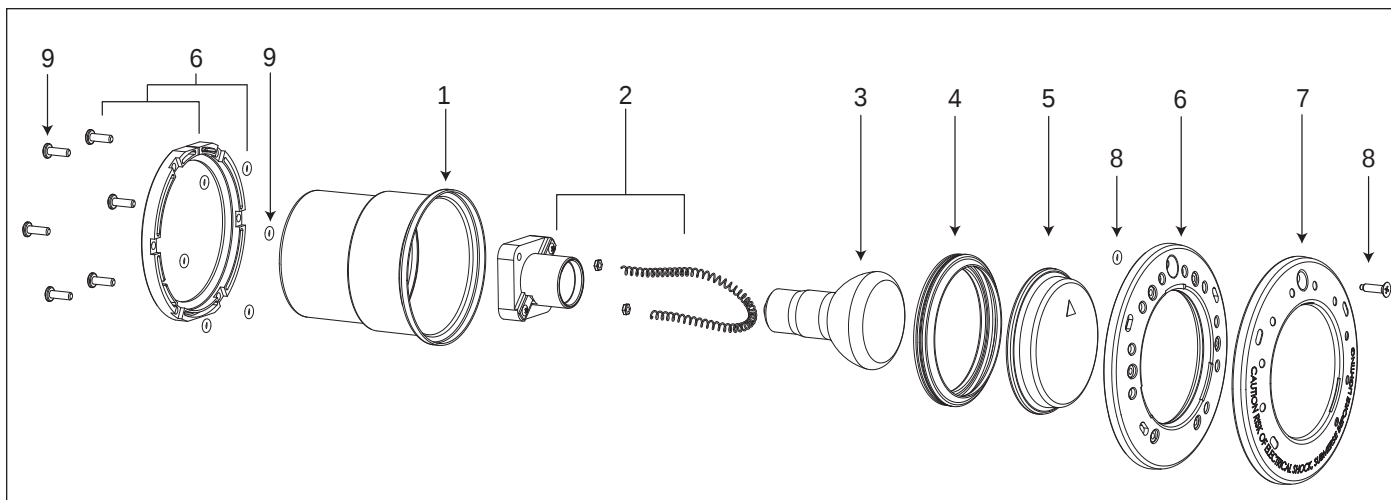
Figure 6. Lampe blanche de spa Jandy, vue éclatée
