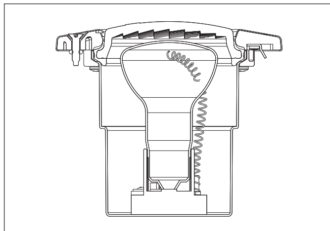
Figure 8. Vue en coupe de la lampe blanche de spa Jandy
