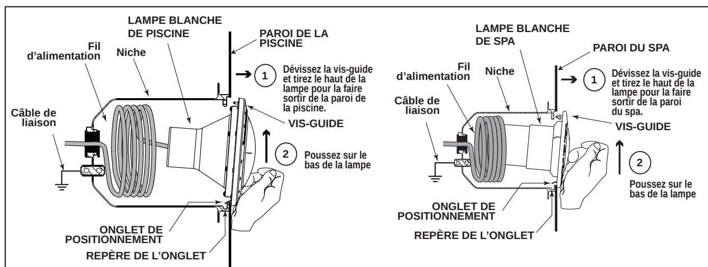
Figure 1. Démontage de la lampe blanche de piscine et de spa pour son remplacement
