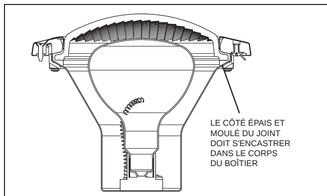
Figure 5. Vue en coupe de la lampe blanche de piscine Jandy
