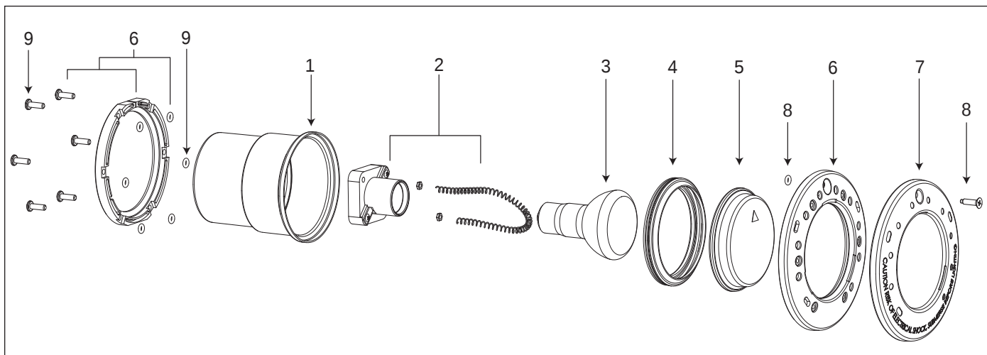
Figura 6. Plano de despiece de la luz blanca Jandy para spas
