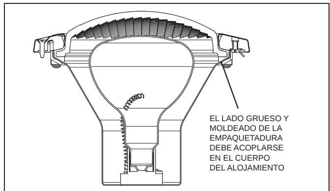
Figura 5. Plano transversal de la luz blanca Jandy para piscinas
