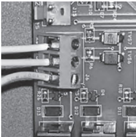
Figura 11A. Conexión remota de Piscina-Apagado-Spa (Conexión de 3 cables)
