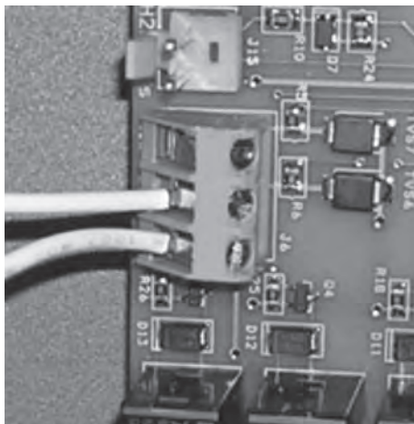
Figure 11b. Connection à AquaLink® RS ou TSTAT à distance (Connexion à 2 fils)
