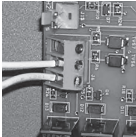
Figura 11B. AquaLink RS o conexión al TSTAT remoto (Conexión de 2 cables)
