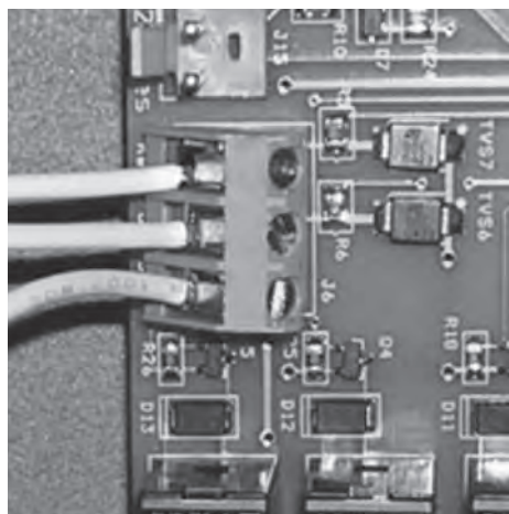
Figure 11a. Connexion à un sélecteur Pool-Off-Spa (Piscine-Arrêt-Spa) à distance (Connexion à 3-fils)
